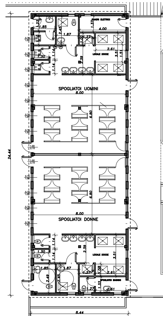
PIANTA SPOGLIATOI
