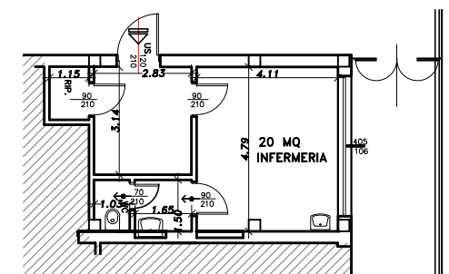
PIANTA INFERMERIA
