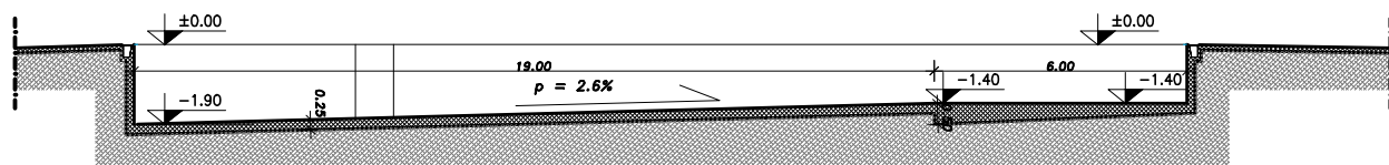
SEZIONE LONGITUDINALE VASCA GRANDE
